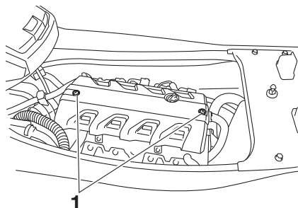
1 Tornillo de la tapa del motor
