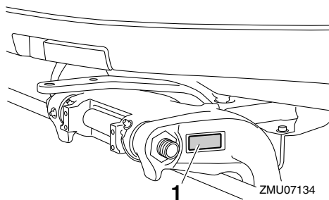
1. Situación del número de serie del motor fueraborda
