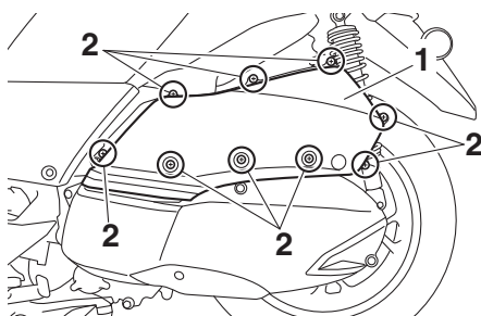
1. Cubierta de la caja del filtro de aire 2. Tornillo
